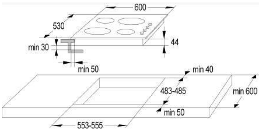
Рис. 1. Подготовка столешницы к монтажу.
